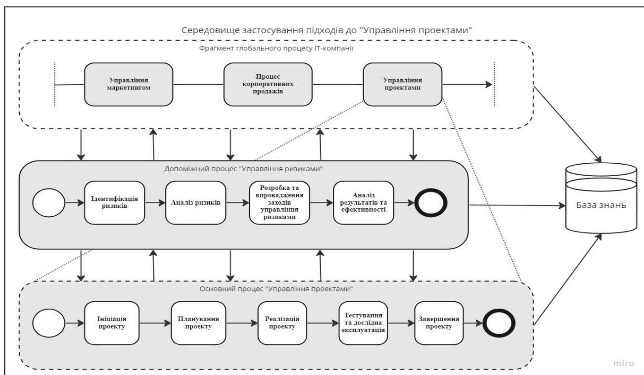
Рис. 1 – Модель зв'язку між бізнес-процесами управління ризиками, IT-проектами, IT-компаніями та їх загальними знаннями.
