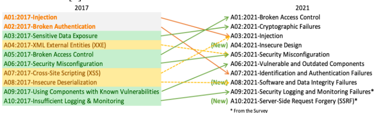
Рис.1. 10 главных угроз безопасности веб-приложений в 2017 и 2021гг [5].
